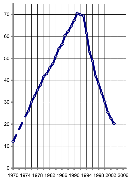
Рис. 8. Потребление электроэнергии на производственные цели в сельскохозяйственных предприятиях РСФСР и РФ, млрд. кВт-ч.
